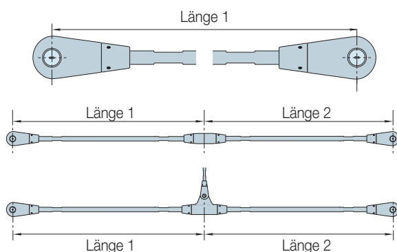
Typ A (ohne Kupplung)
