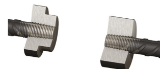
Ancon-TTH Endverankerung 1 Gewinde, 1 TTH Endverankerung montiert
